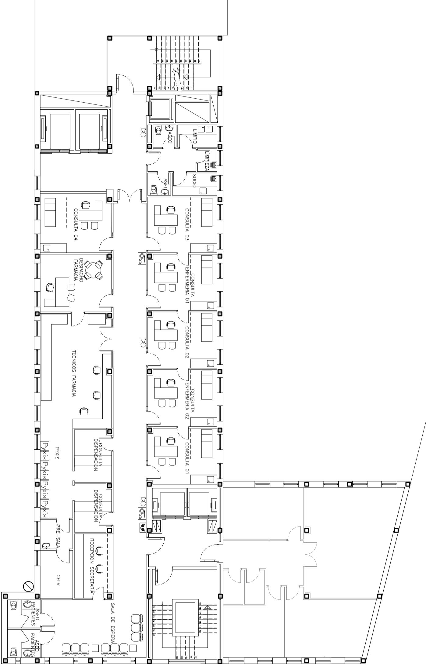
PLANTA SEXTA
